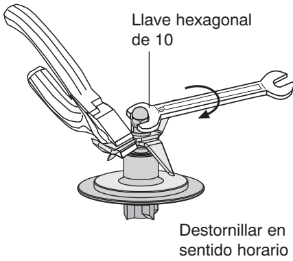
Desmontaje cuchilla
