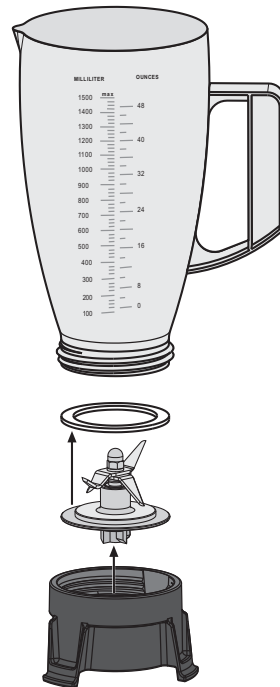
Remoción del bloque cuchillas
