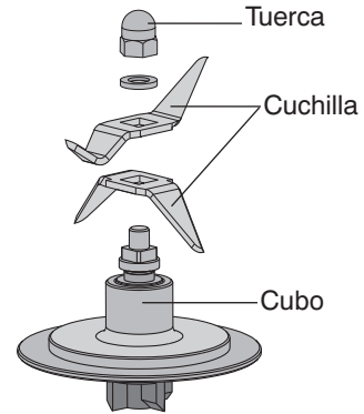
Elementos bloque cuchilla
